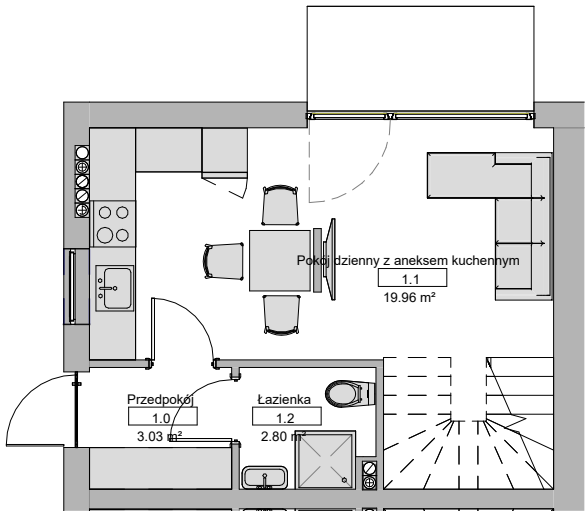
RZUT PARTERU 1:100
