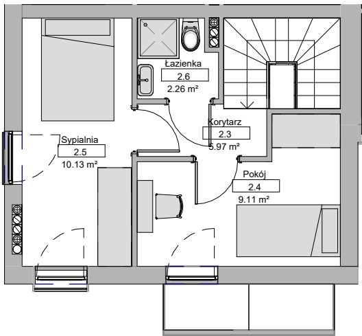
RZUT I PIĘTRA 1:100
