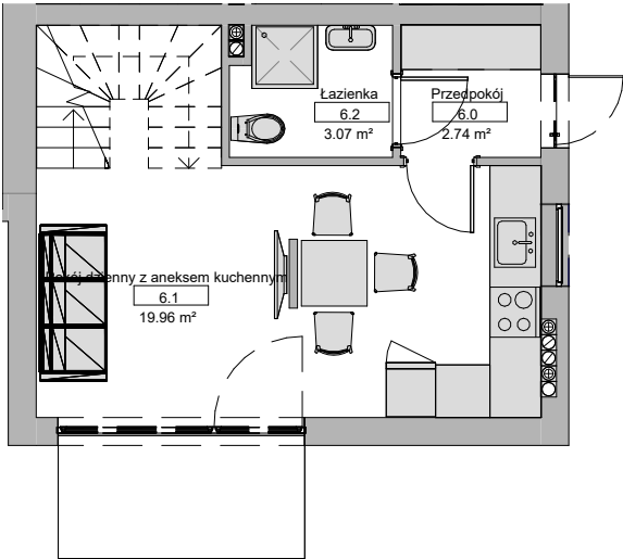
RZUT PARTERU 1:100
