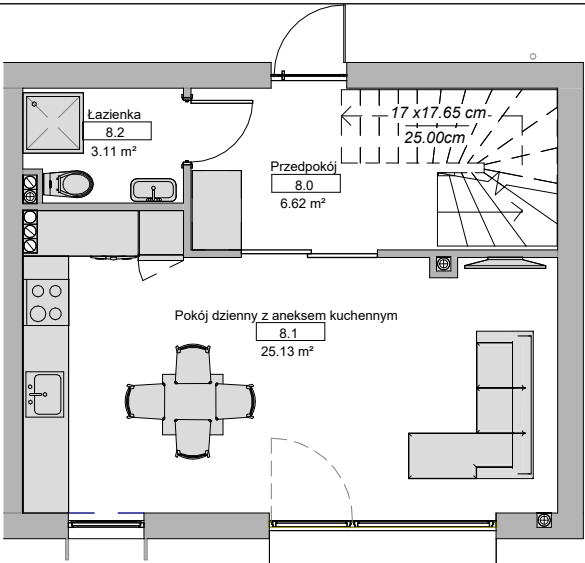
RZUT PARTERU 1:100
